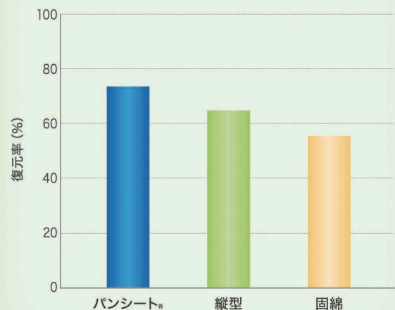
圧縮残留ひずみ試験
