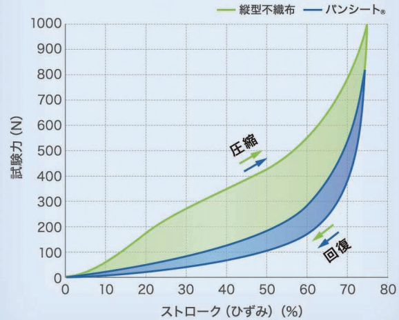
圧縮/回復曲線
